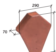
Ukončení hřebenače univerzální Réf. 801
