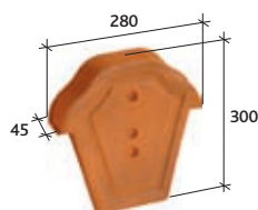
Ukončení hřebenače Losangée Réf. 809
