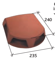
Klobouk prostupové tašky Ø 120 mm a 150 mm (130 cm²) Réf. 1000
