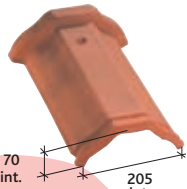
Hřebenač Losangée (2,5 ks / bm) Réf. 716
