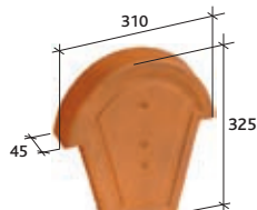
Ukončení hřebenače Réf. 807
