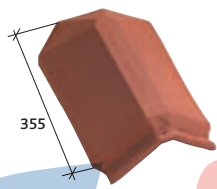
Koncový hřebenač Réf. 859
